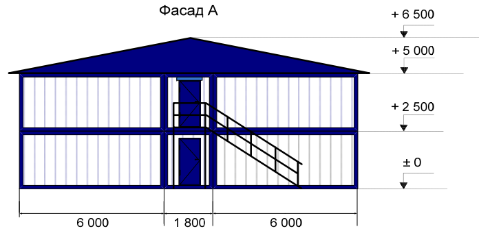
Фасад А
