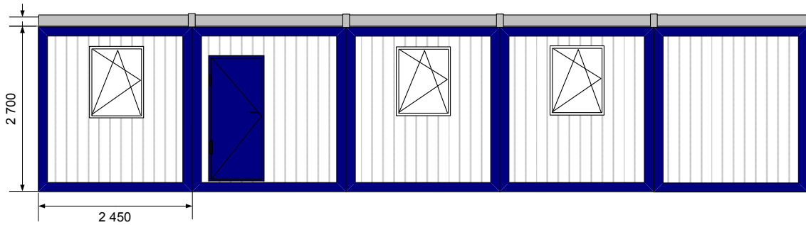
Фасад
