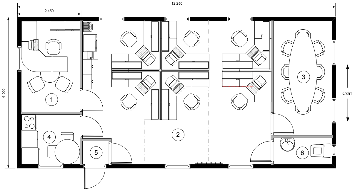
Планировка
